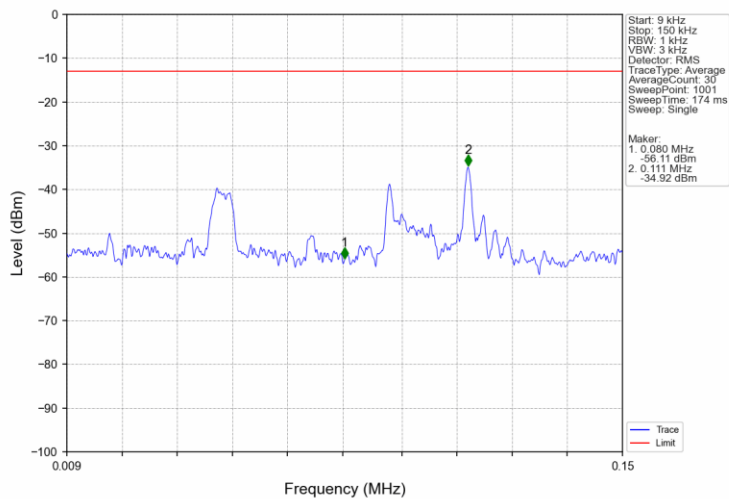
Band66_20MHz_16QAM_LCH_1720MHz_RB_1_0_NTNV
