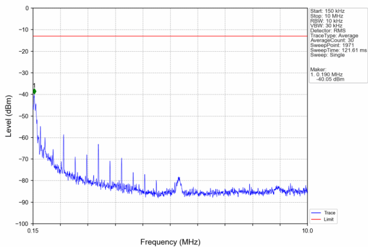
Band66_20MHz_16QAM_LCH_1720MHz_RB_1_0_NTNV
