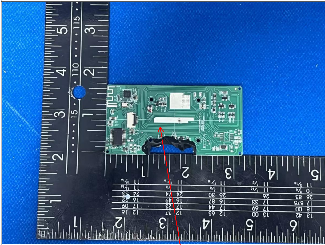
NFC Antenna
