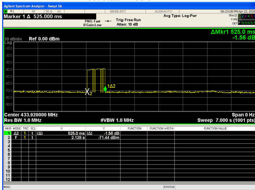
Test data—433.92MHz
