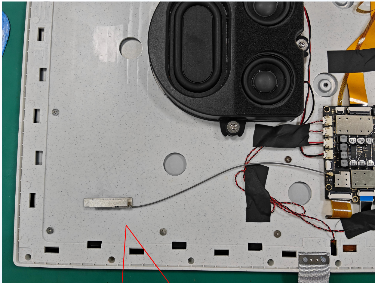
WIFI/BT天线
