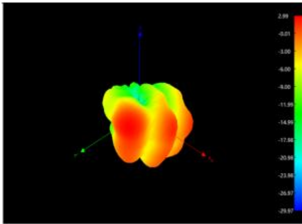
2480Mhz
