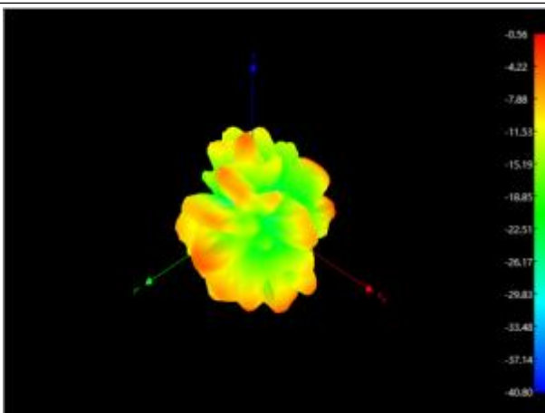
WiFi: 5350Mhz
