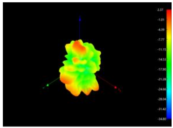
WiFi: 5150Mhz
