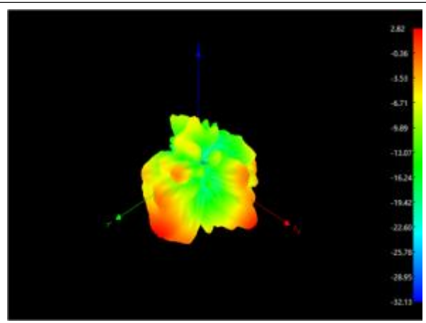
WiFi: 5850Mhz
