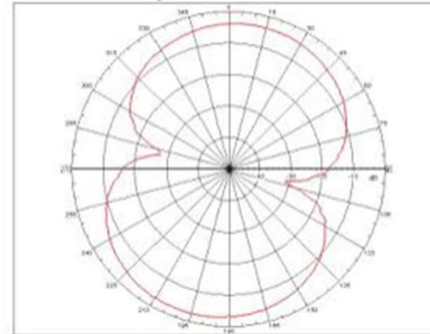
E-PLANE
