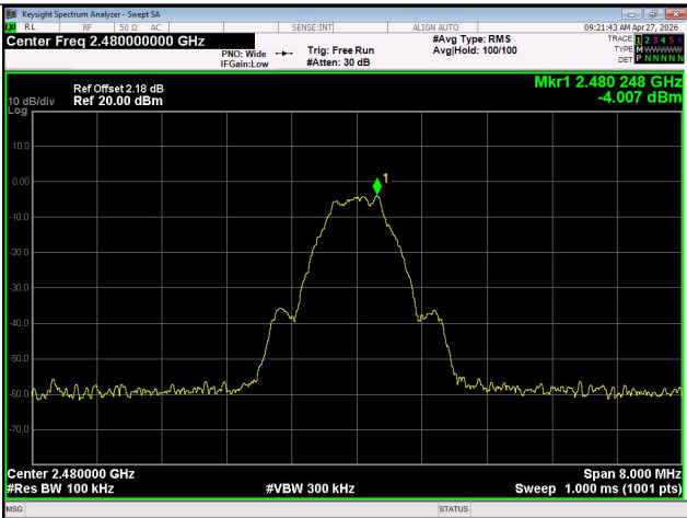
BLE 1M: Band Edge, Right Side
