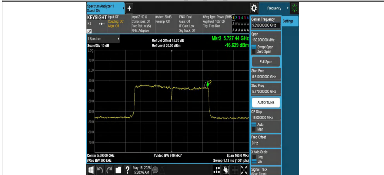
11AC80MIMO_Ant2_5690_UNII-3
