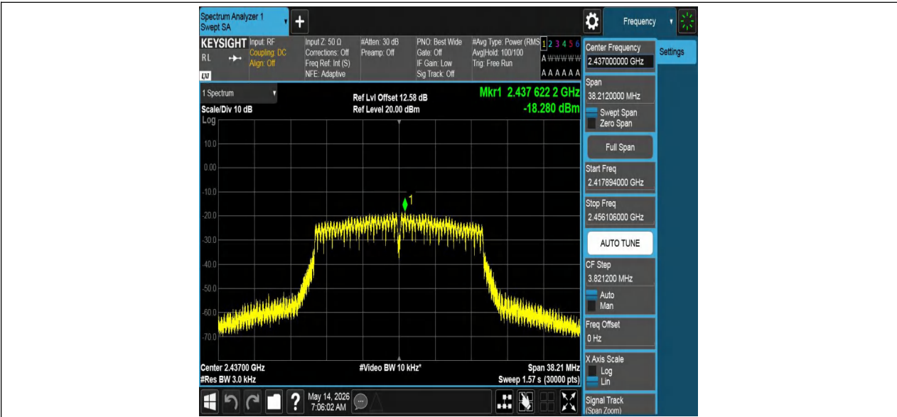
11N20MIMO_Ant2_2437
