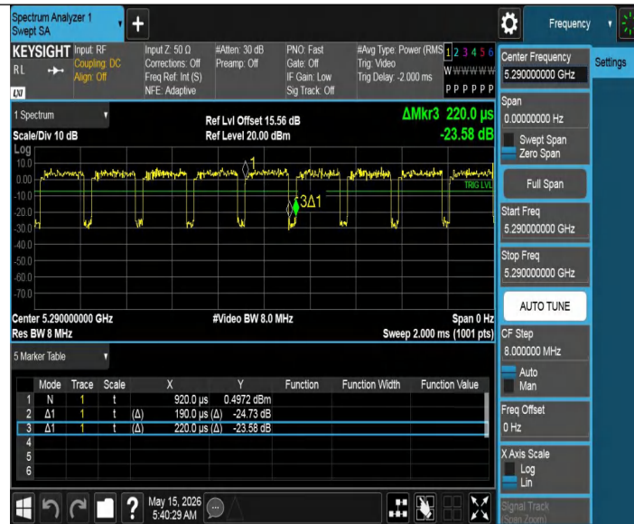
11AC80MIMO_Ant2_5290
