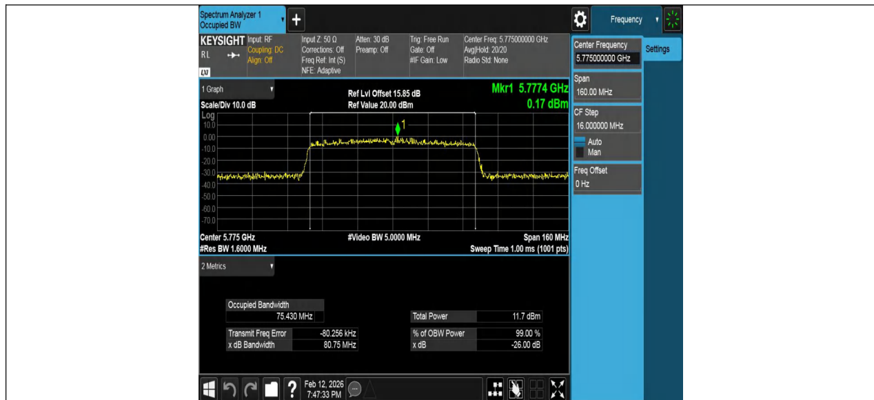
11AC80MIMO_Ant2_5775
