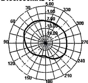
2400.000MHz H
