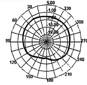
2500.000MHz H
