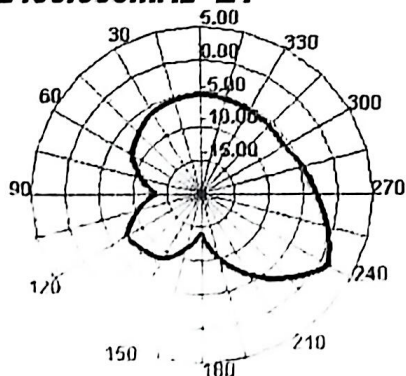
2400.000MHz E1
