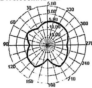
2400.000MHz E2
