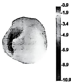
2400.000MHz E1
