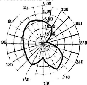
2400.000MHz E1
