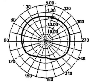
2500.000MHz H
