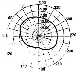
2400.000MHz H
