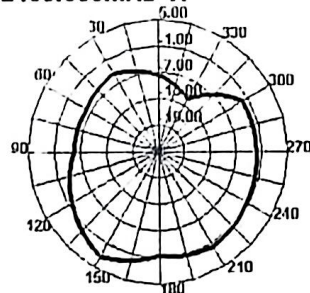
2450.000MHz H
