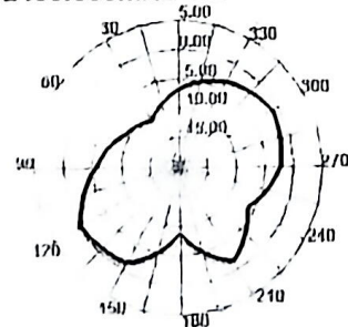
2450.000MHz E2
