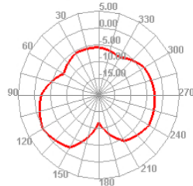
2450.000MHz E2
