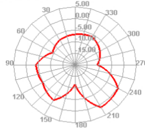
2400.000MHz E1
