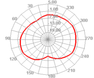
2400.000MHz H
