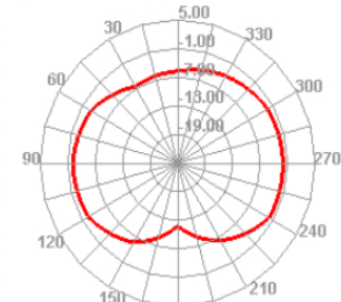
2500.000MHz H
