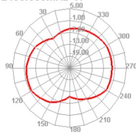
2450.000MHz H
