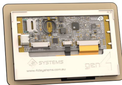
gen4-ESP32-43CT-CLB Rear
