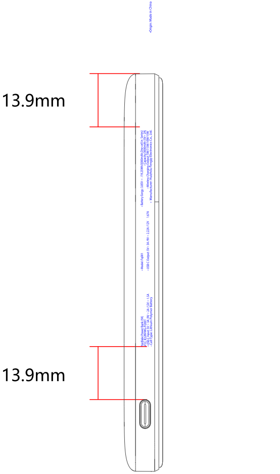
磁吸充电宝右视图
