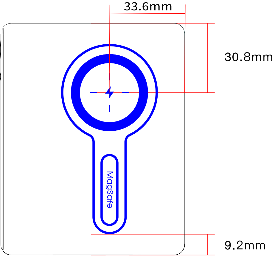
大容量充电宝后视图
