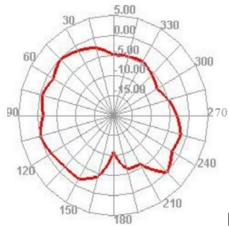
2465.000MHz E2
