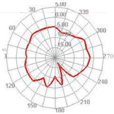
2465.000MHz E1
