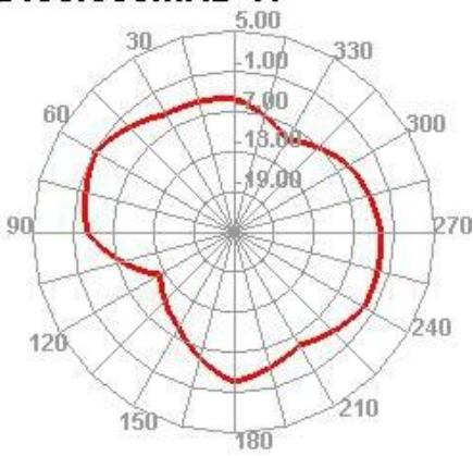
2450.000MHz H
