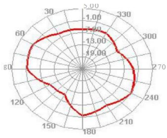
2465.000MHz E2
