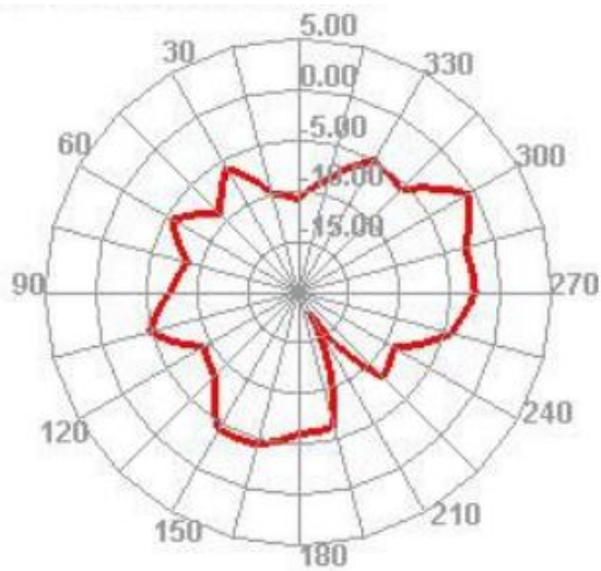
2415.000MHz E1
