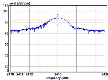
2.4G_SRD_LOW_TX_Horizontal
