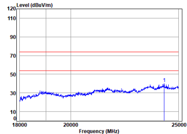
2.4G_SRD_TX_LOW_Horizontal
