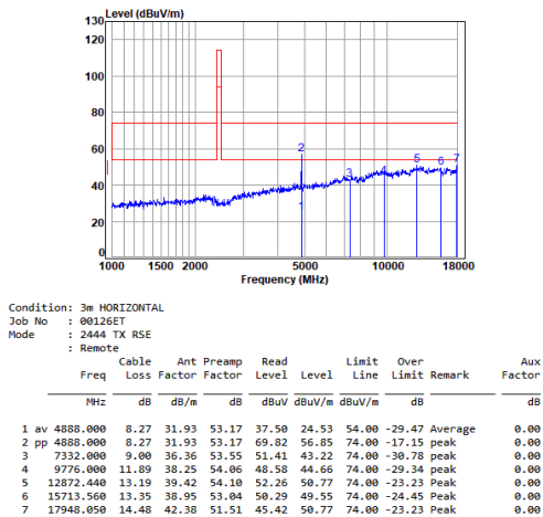
2.4G_SRD_TX_LOW_Horizontal
