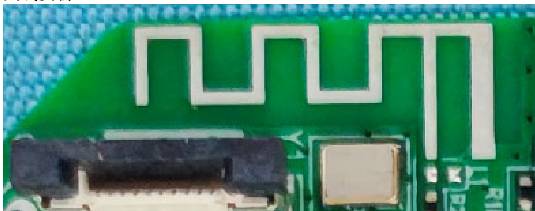
天线实物
