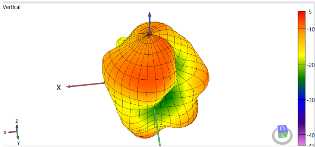
天线 2440MHz 3D-Vertical Pattern
