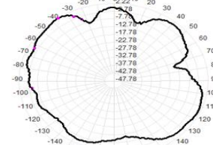
2400.0MHz Total(E1), Max= 2.22dBi
