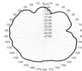
2470.0MHz Total(E1), Max= 3.39dBi
