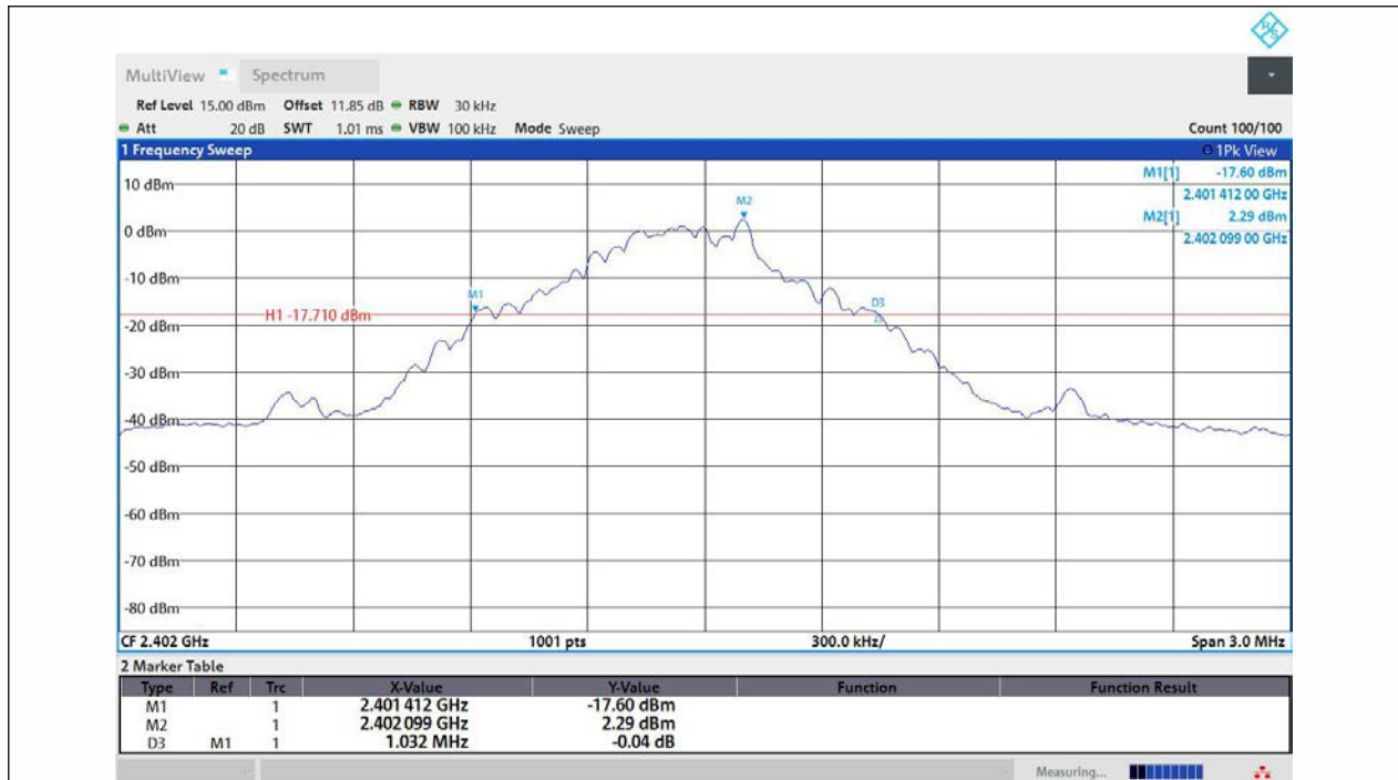
DH5-Ant1-2402
