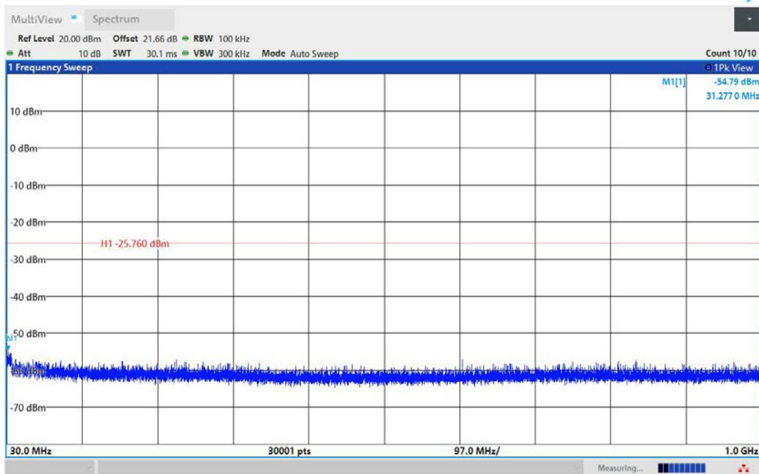
11G-Ant1-2437-30~1000-PASS
