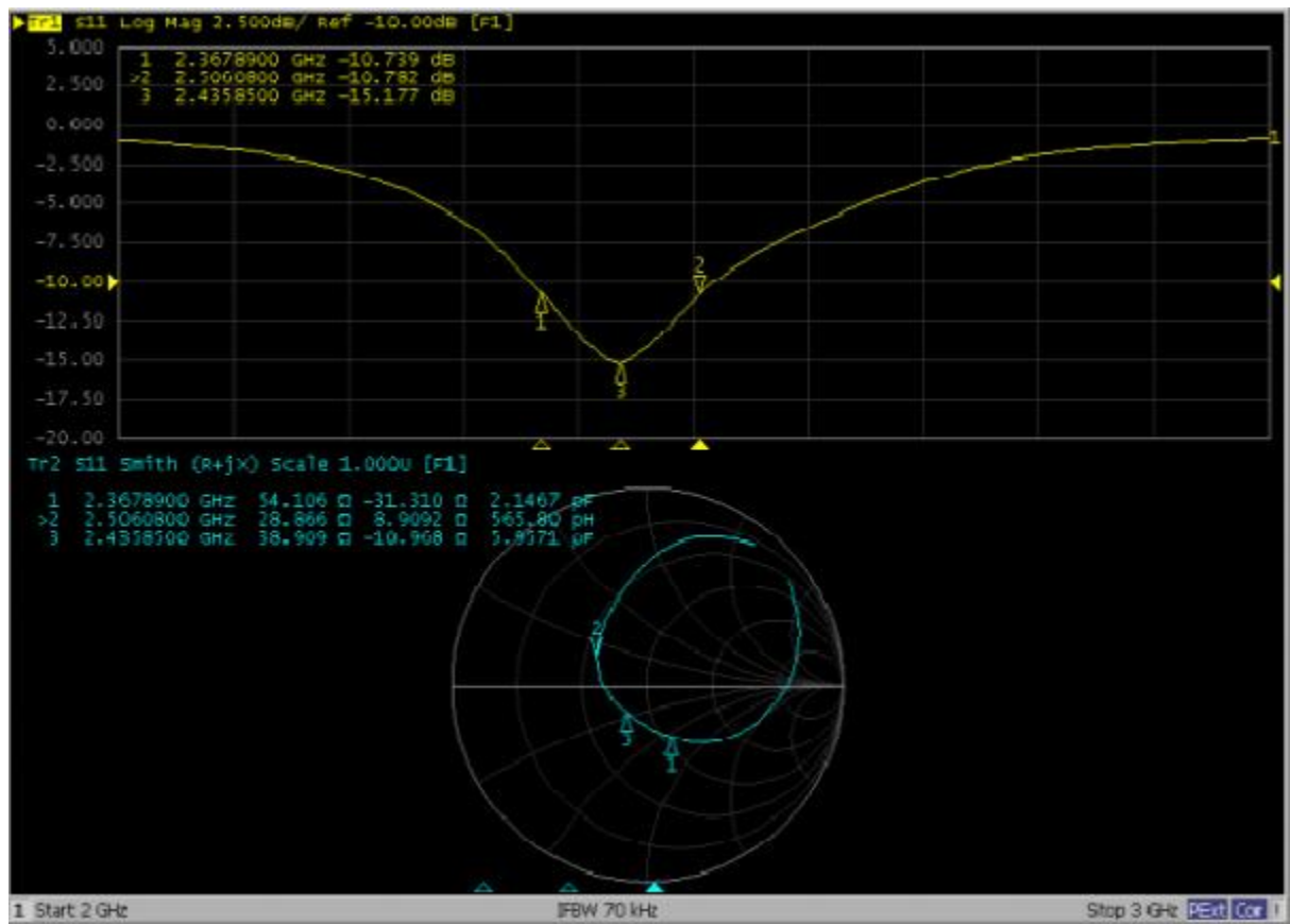
Fig. 2 Normal Module PIFA Antenna S11
