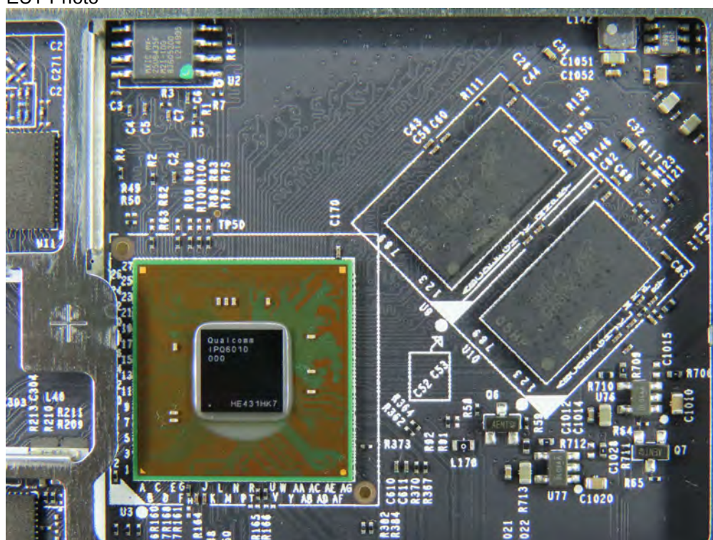
(60) EUT Photo
