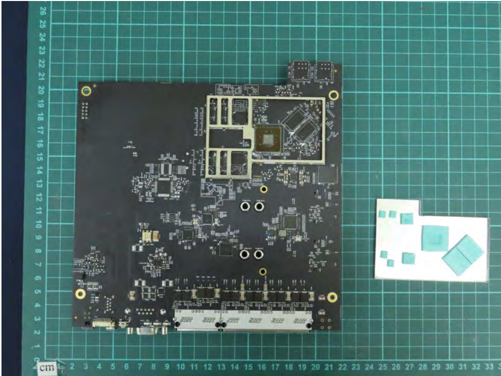
(81) EUT Photo
