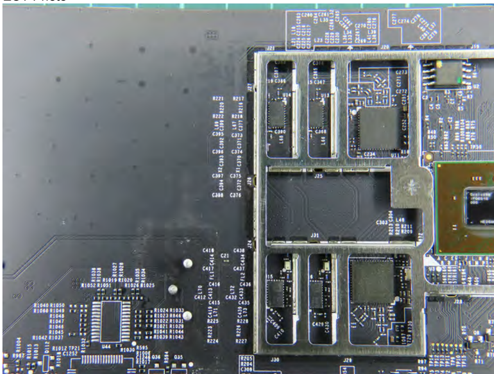
(85) EUT Photo
