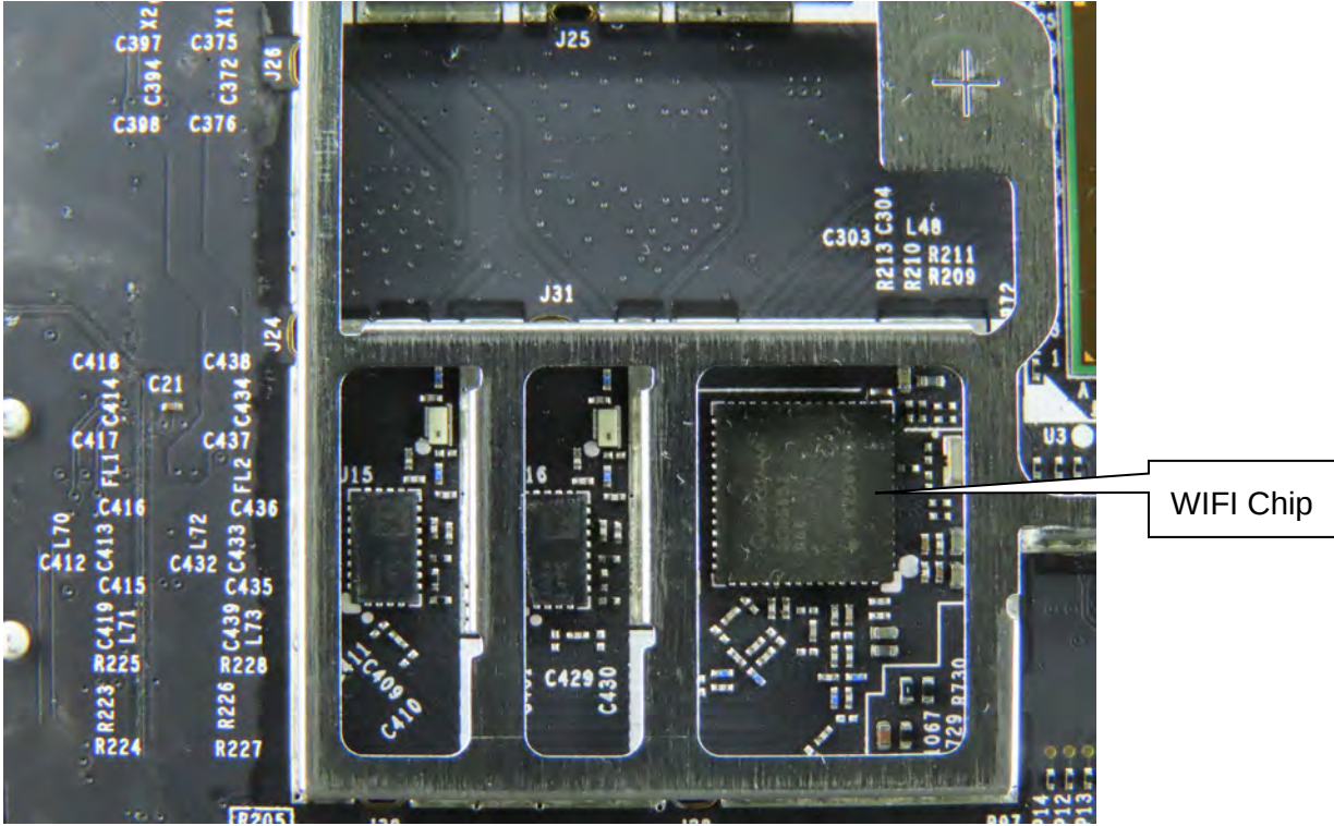
(87) EUT Photo
