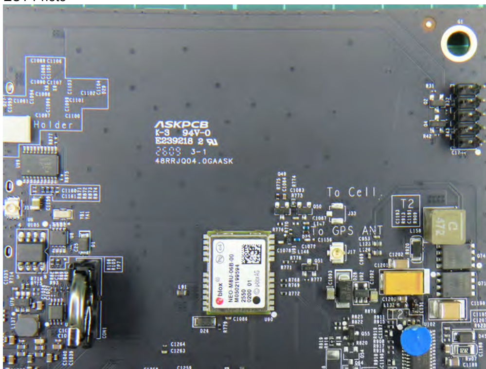
(77) EUT Photo
