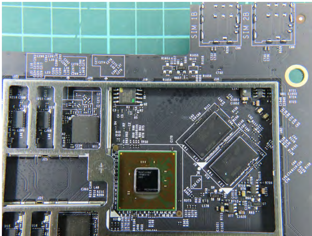
(91) EUT Photo
