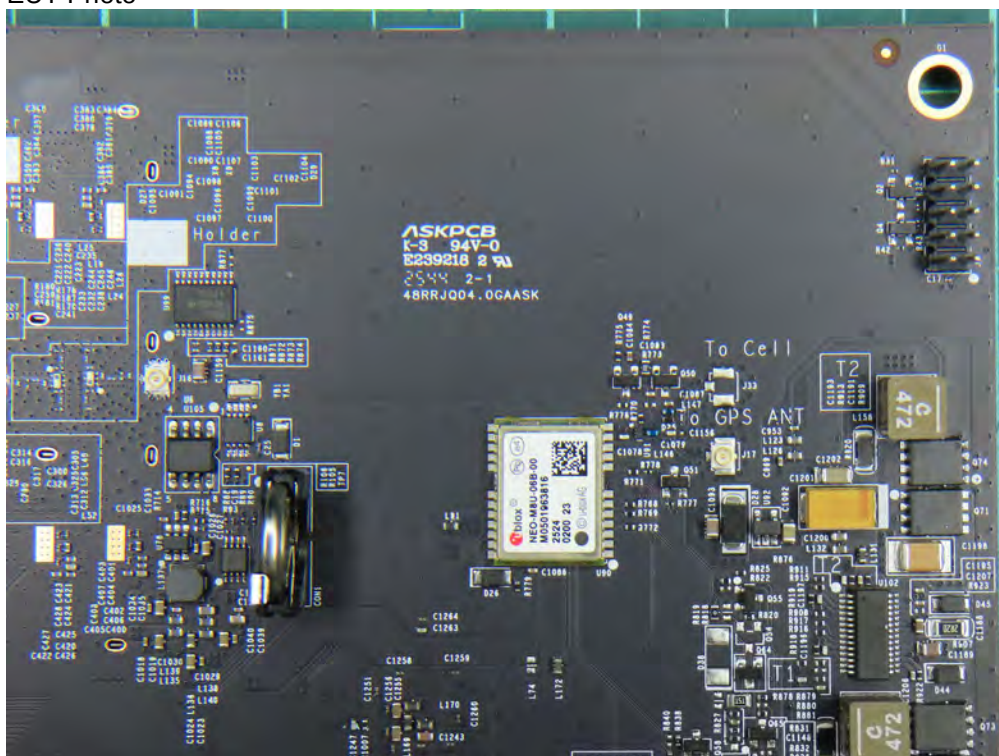
(48) EUT Photo
