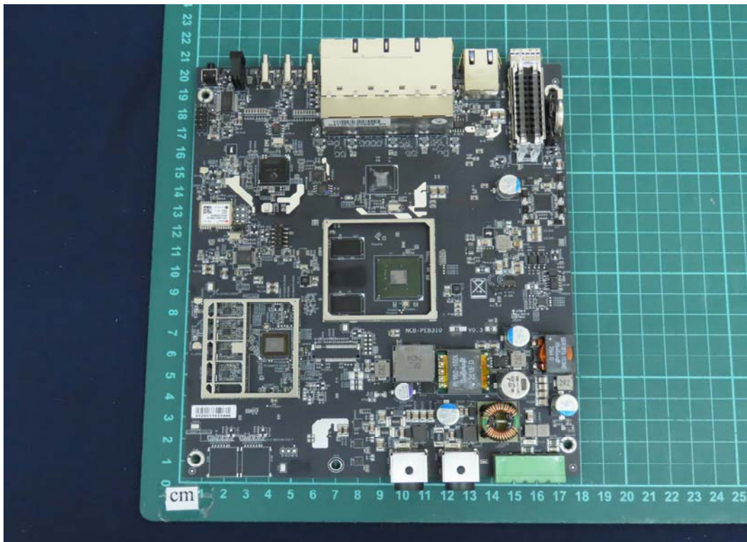
(48) EUT Photo
