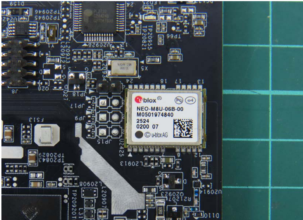
(40) EUT Photo
