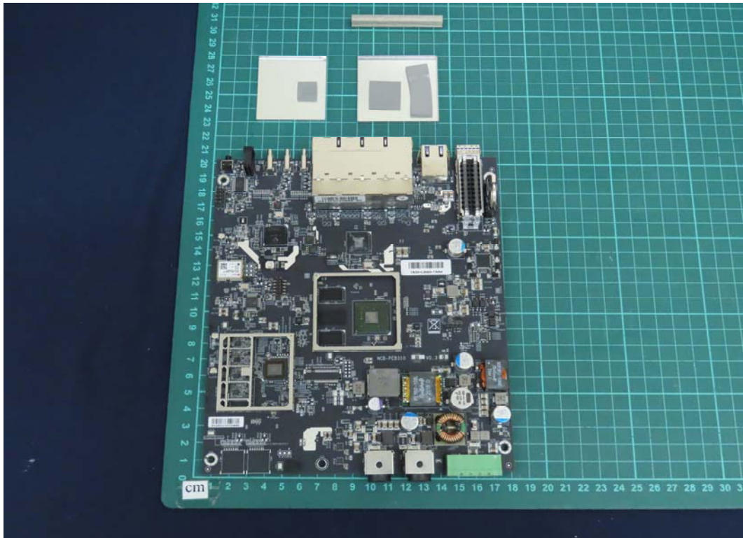
(48) EUT Photo
