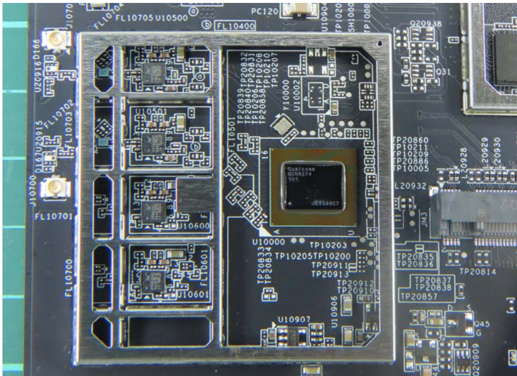
(40) EUT Photo
