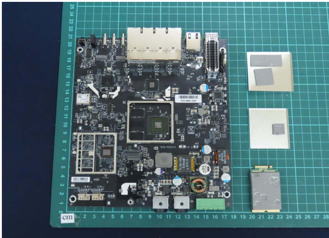
(36) EUT Photo
