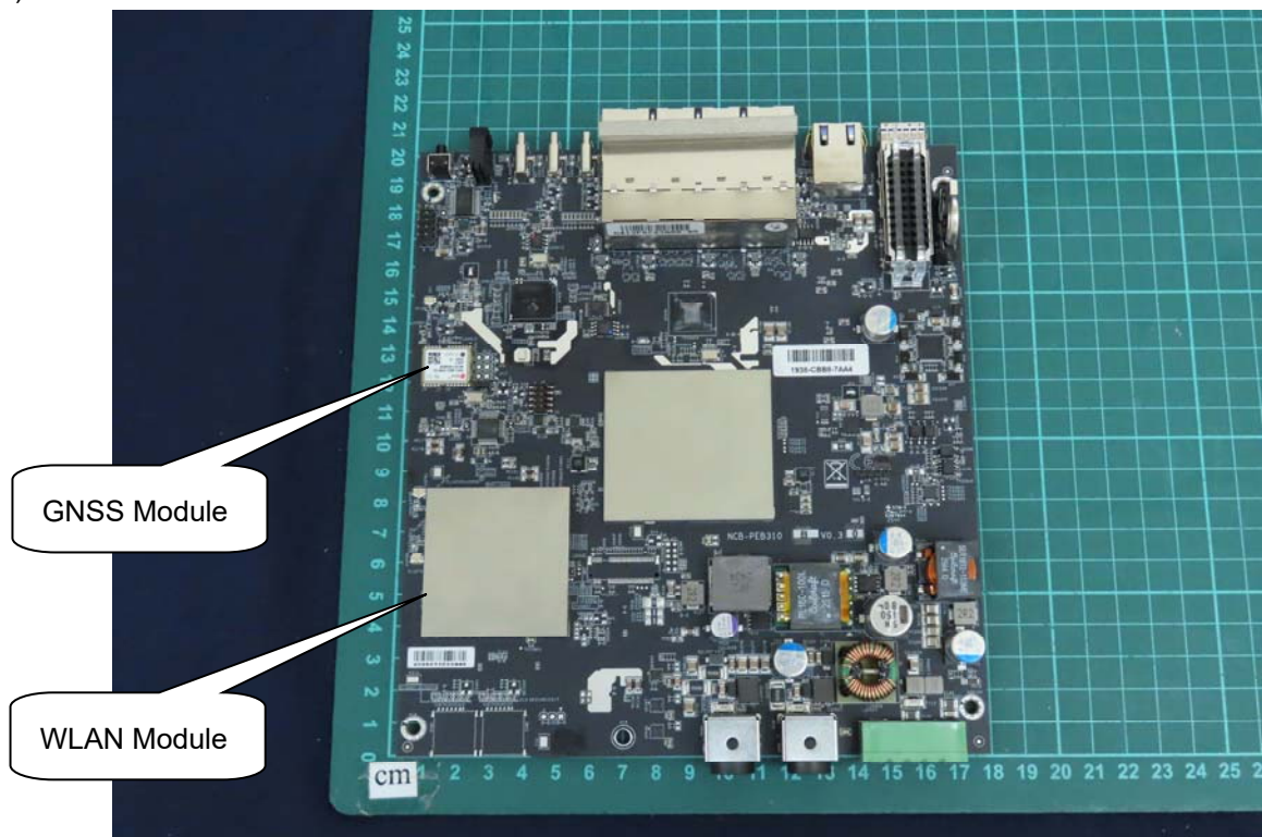
(46) EUT Photo
