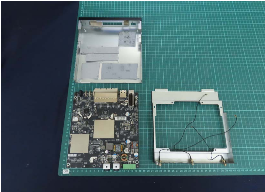
(46) EUT Photo
