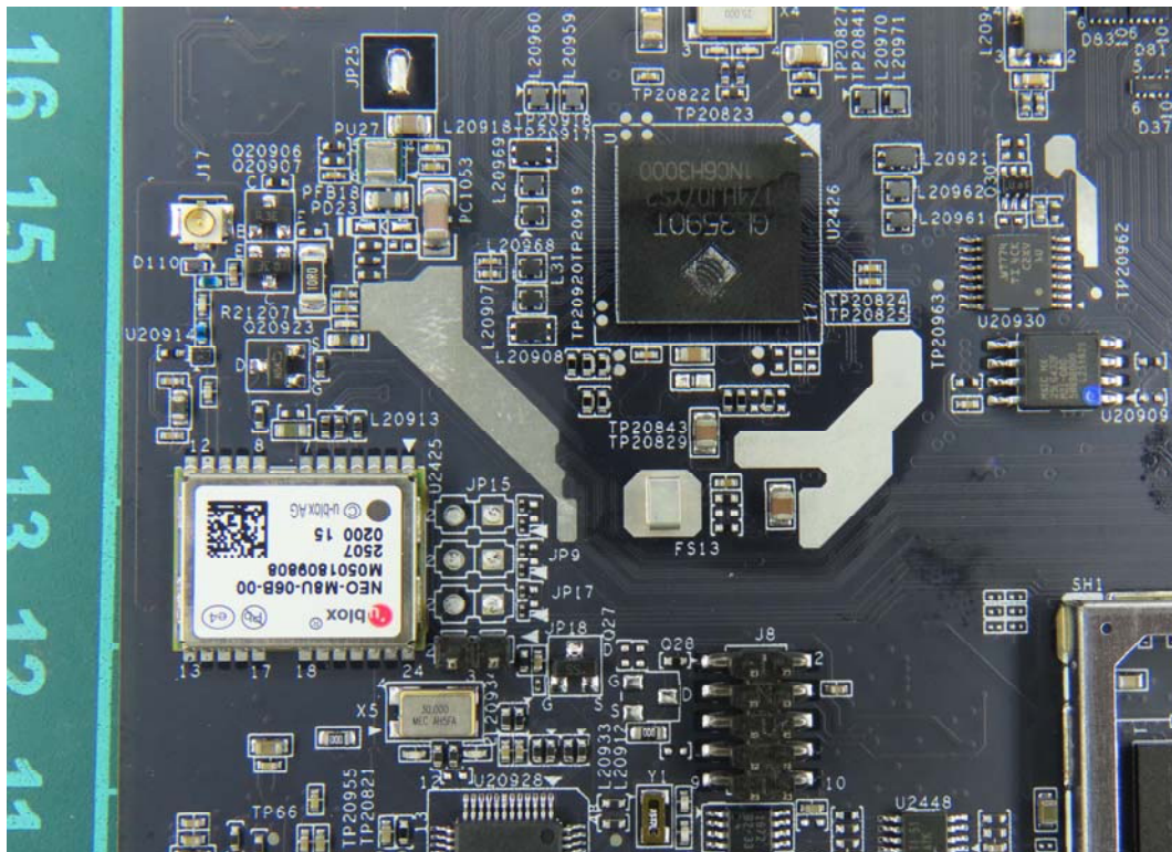
(50) EUT Photo
