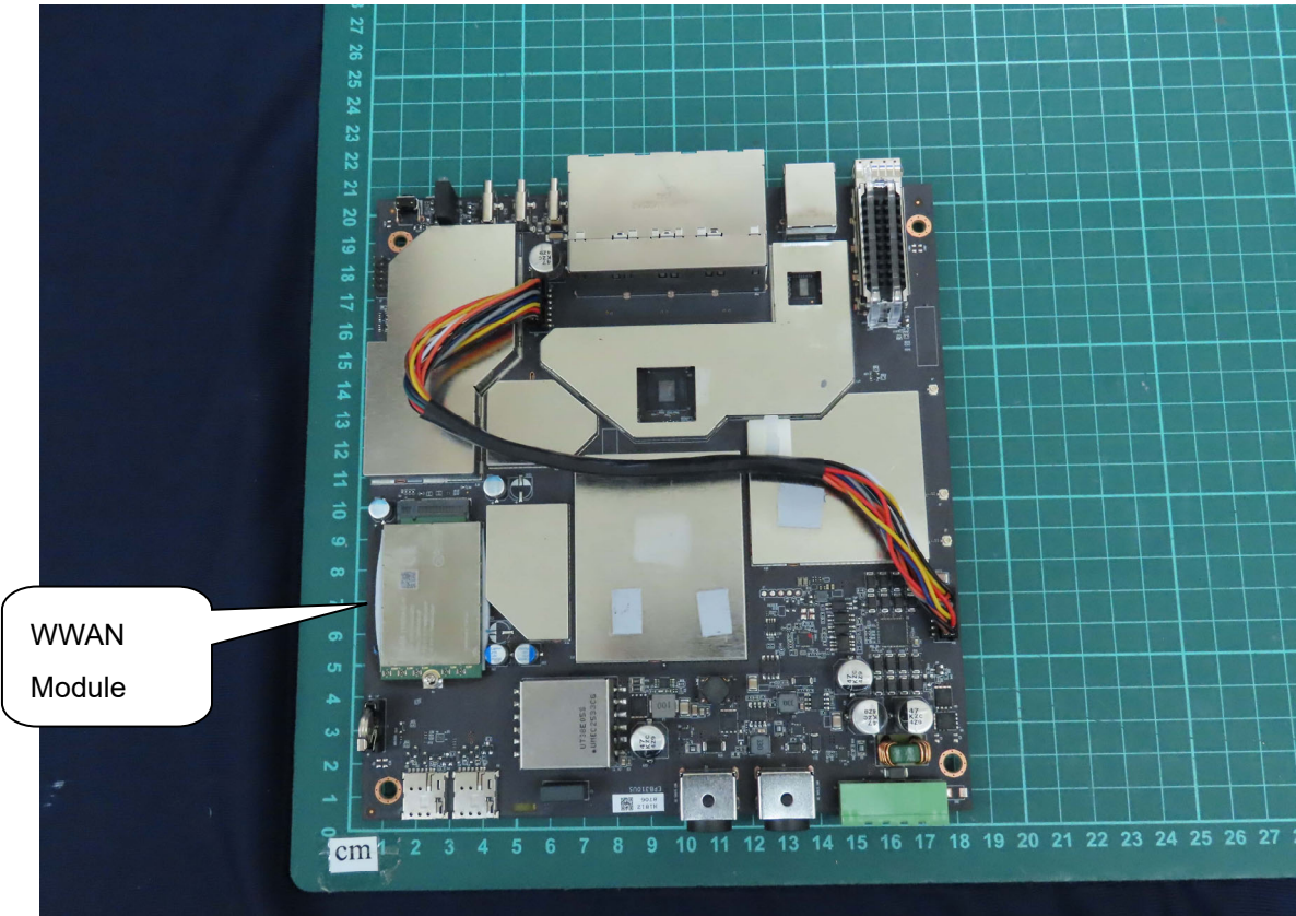
(20) EUT Photo
