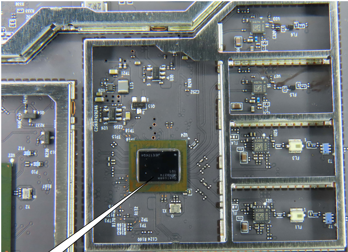
(24) EUT Photo
