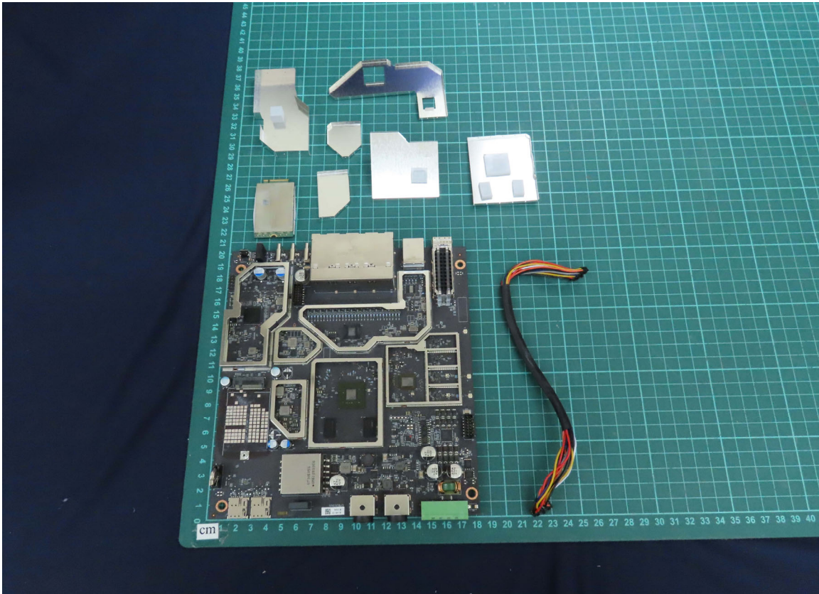
(21) EUT Photo
