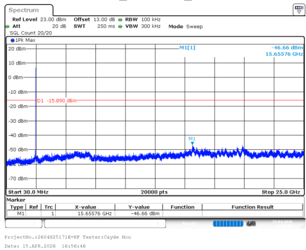
802.11b_2462MHz_Chain 1
