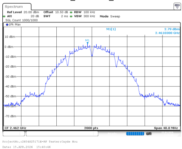
802.11b_2462MHz_Chain 0
