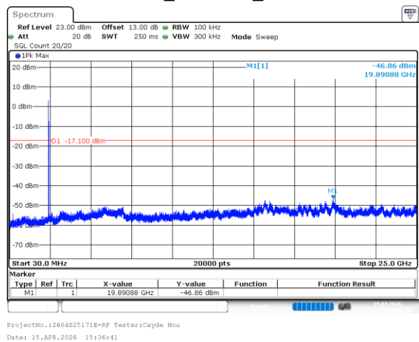
802.11b_2437MHz_Chain 0
