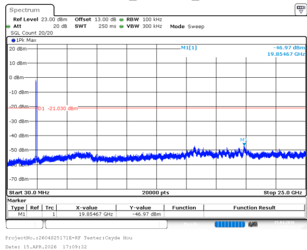
802.11n20_2437MHz_Chain 1
