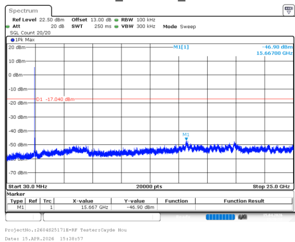
802.11b_2437MHz_Chain 0
