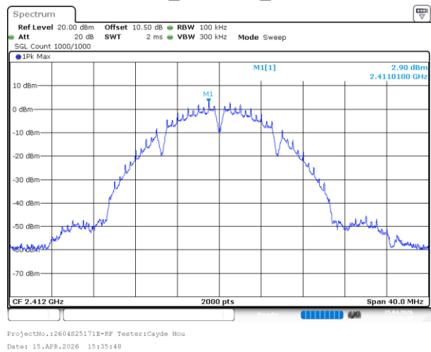
802.11b_2412MHz_Chain 0
