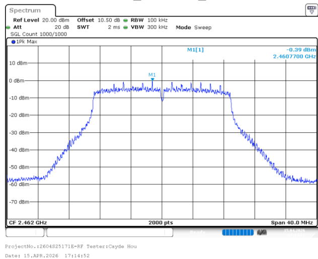
802.11n20_2462MHz_Chain 1
