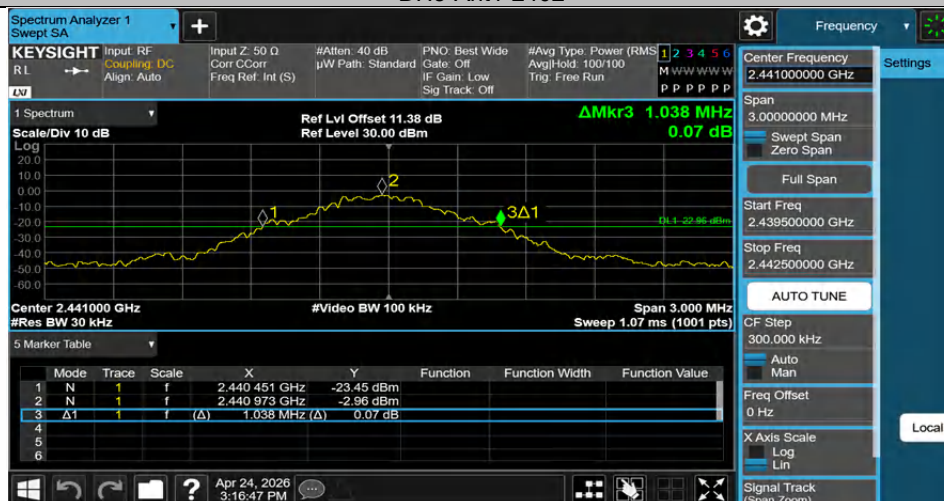
DH5-Ant1-2441
