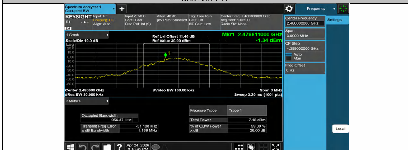
DH5-Ant1-2480
