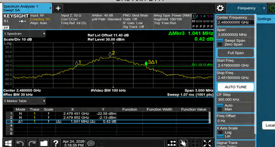
DH5-Ant1-2480
