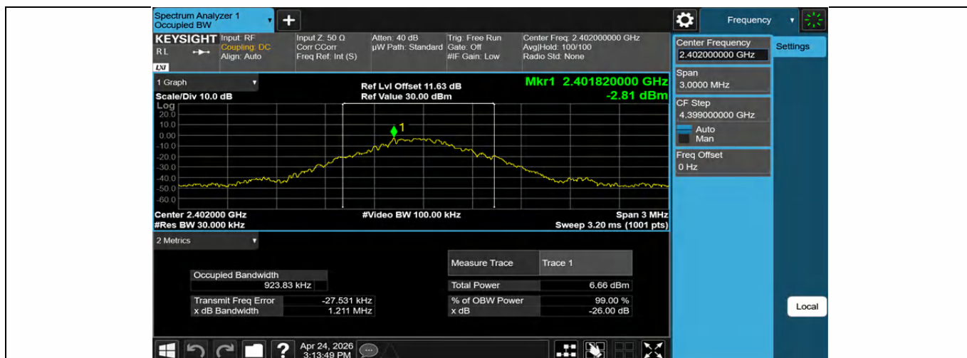
DH5-Ant1-2402
