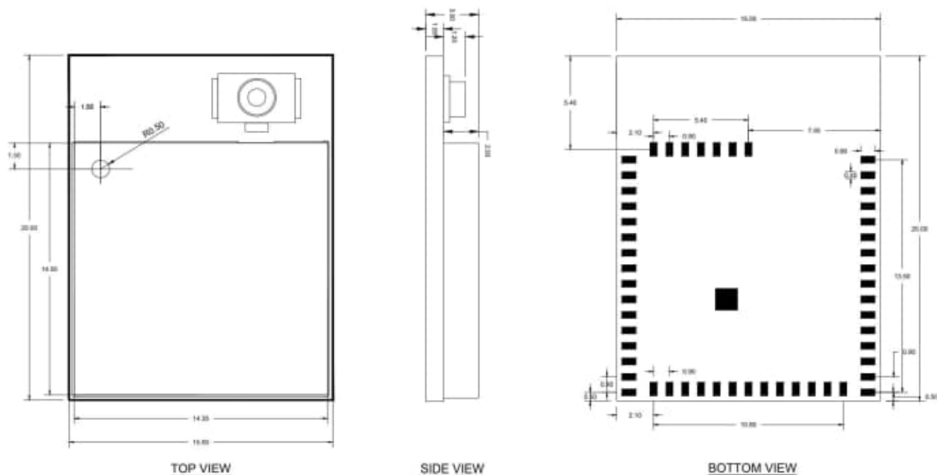
Figure 23. RRQ61001-009 module dimensions
