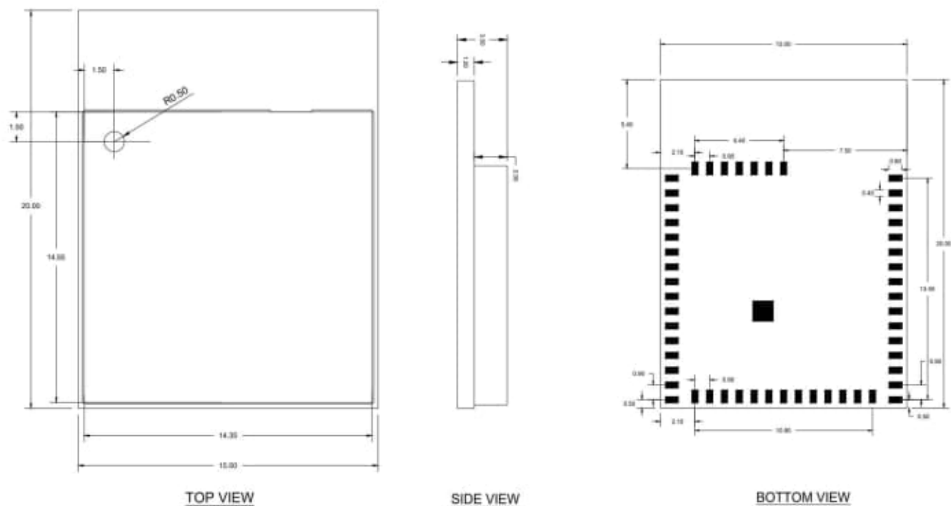
Figure 24. RRQ61001-008 module dimensions
