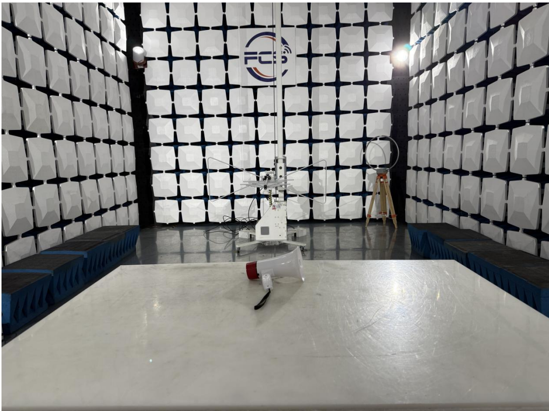
RE (Below1GHz)
