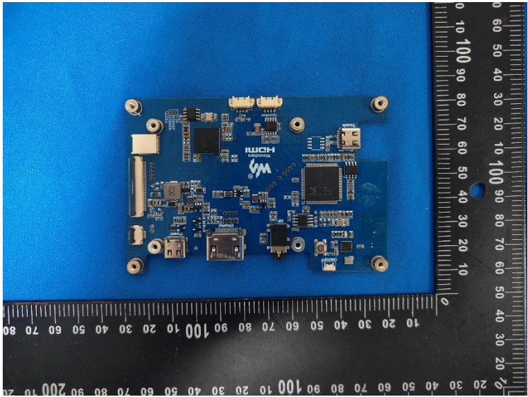
BLE Antenna
