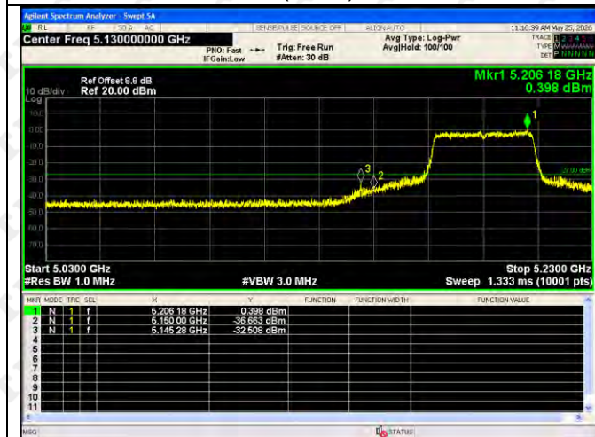
802.11ac(VHT80)-5210
