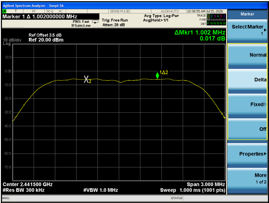
\pi/4 -DQPSK mode-CH39
