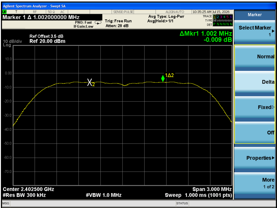
\pi/4 -DQPSK mode-CH00
