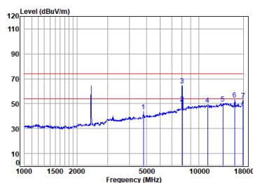
11b_TX_CH_01_Horizontal
