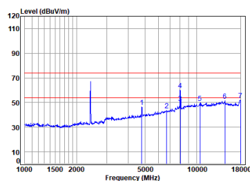
11b_TX_CH_01_Vertical
