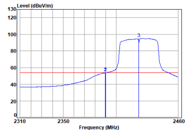
11n_HT(40M)_TX_CH_03_Vertical-Avg
