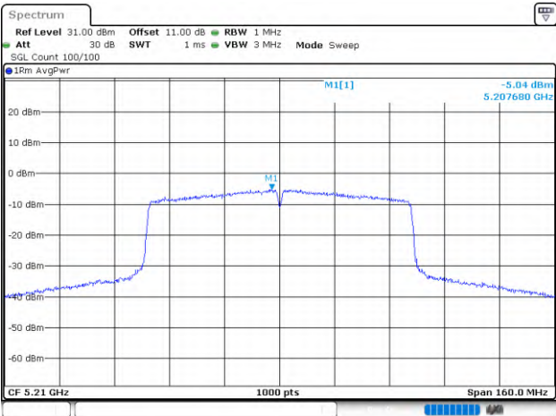
802.11ac80_5210MHz_Chain 1
