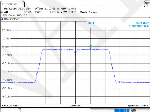
802.11ac40_5230MHz_Chain 1
