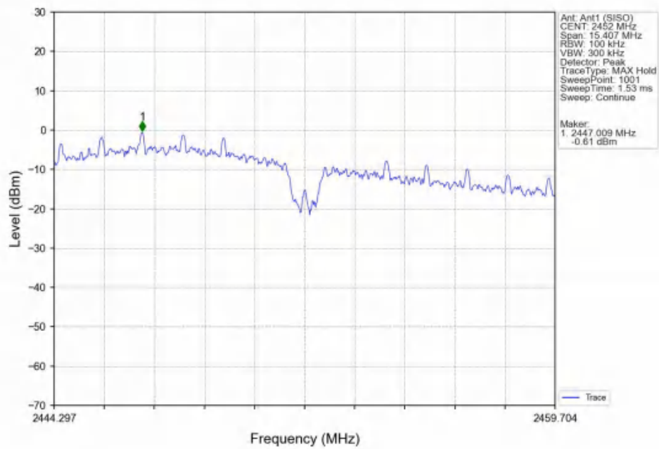
802.11ax(HEW40)_HCH_2452MHz_SU_/_Ant1 (SISO)_NTNV
