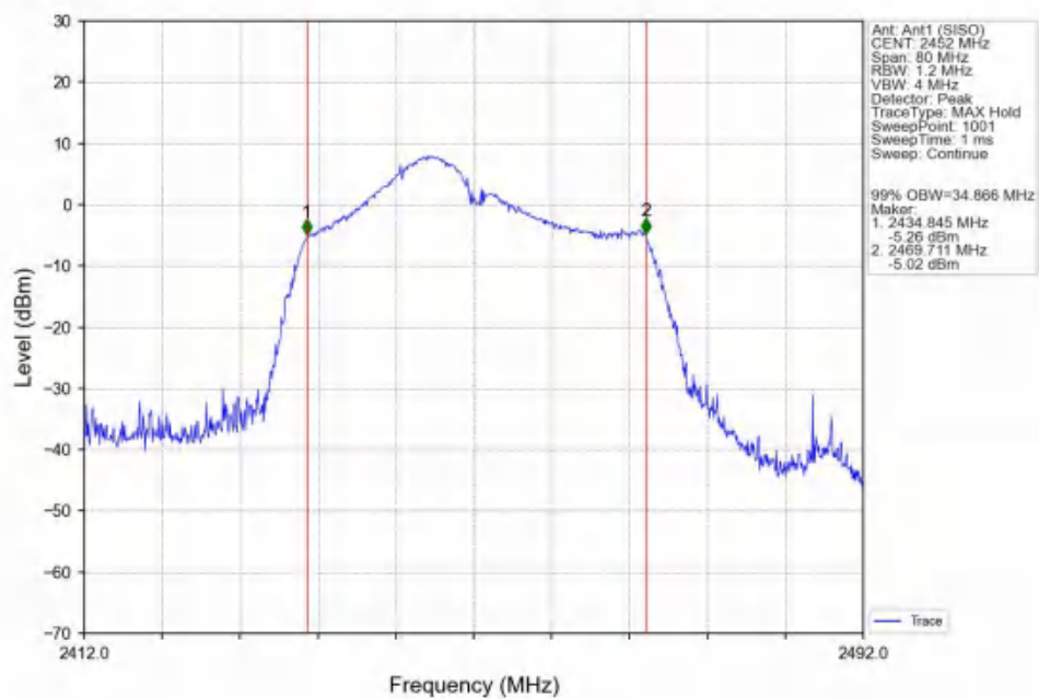
802.11ax(HEW40)_HCH_2452MHz_SU_/_Ant1 (SISO)_NTNV
