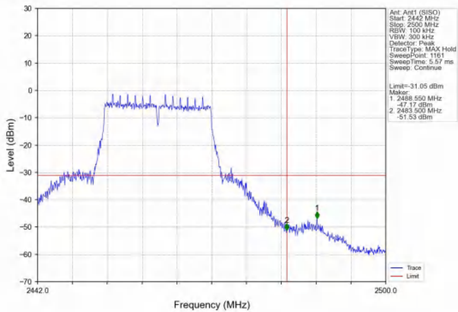
802.11ax(HEW20)_HCH_2462MHz_SU_/_Ant1 (SISO)_NTNV
