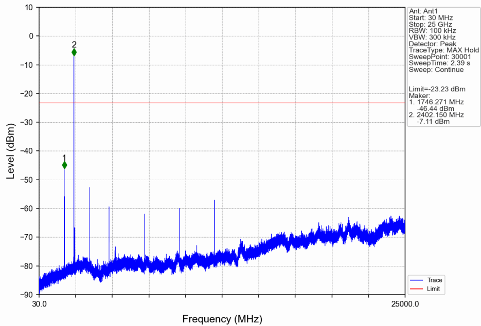
GFSK DH5 LCH 2402MHz Ant1 NTN
