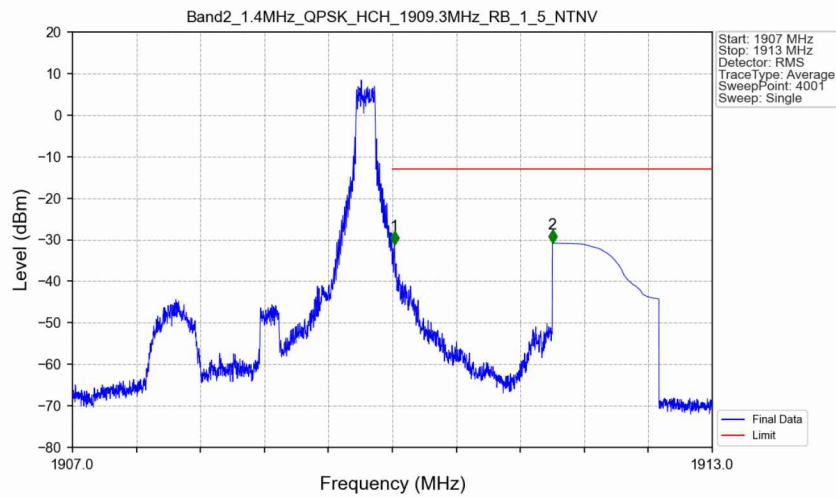
Band2_1.4MHz_QPSK_HCH_1909.3MHz_RB_1_5_NTNV
