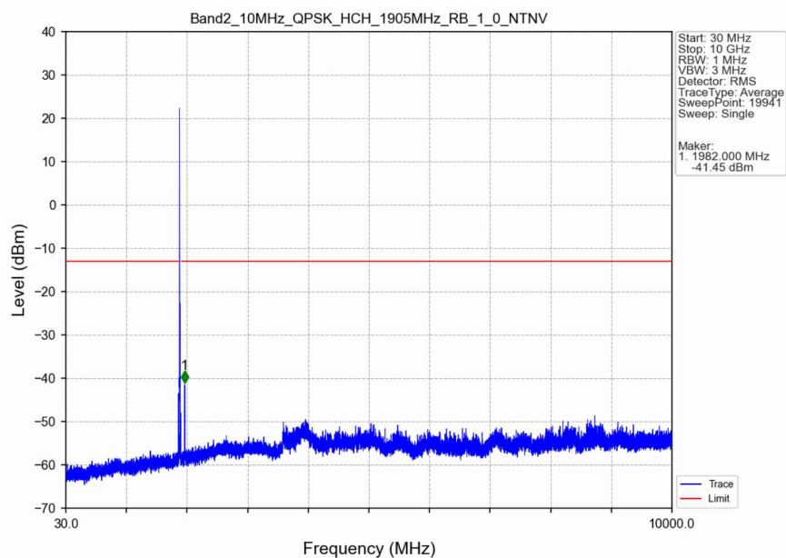
Band2_10MHz_QPSK_HCH_1905MHz_RB_1_0_NTNV
