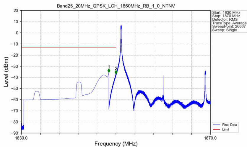
Band25_20MHz_QPSK_LCH_1860MHz_RB_1_0_NTNV
