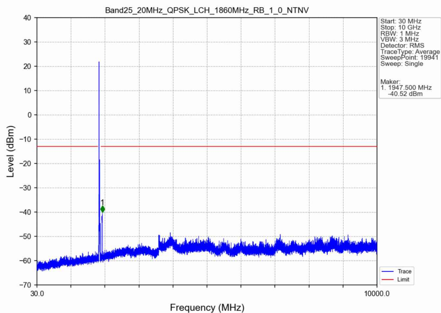
Band25_20MHz_QPSK_LCH_1860MHz_RB_1_0_NTNV
