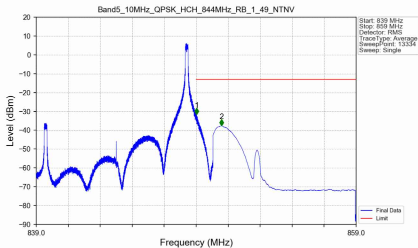
Band5_10MHz_QPSK_HCH_844MHz_RB_1_49_NTNV
