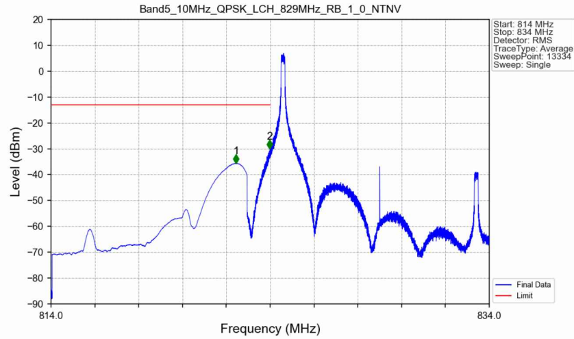
Band5_10MHz_QPSK_LCH_829MHz_RB_1_0_NTNV
