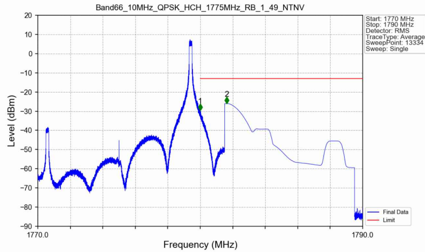
Band66_10MHz_QPSK_HCH_1775MHz_RB_1_49_NTNV
