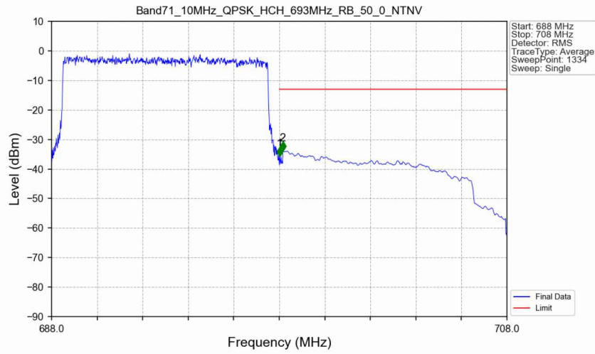
Band71_10MHz_QPSK_HCH_693MHz_RB_50_0_NTNV
