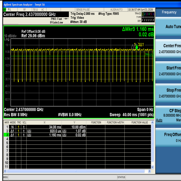
NTNV-11N40MIMO-Ant1-2437
