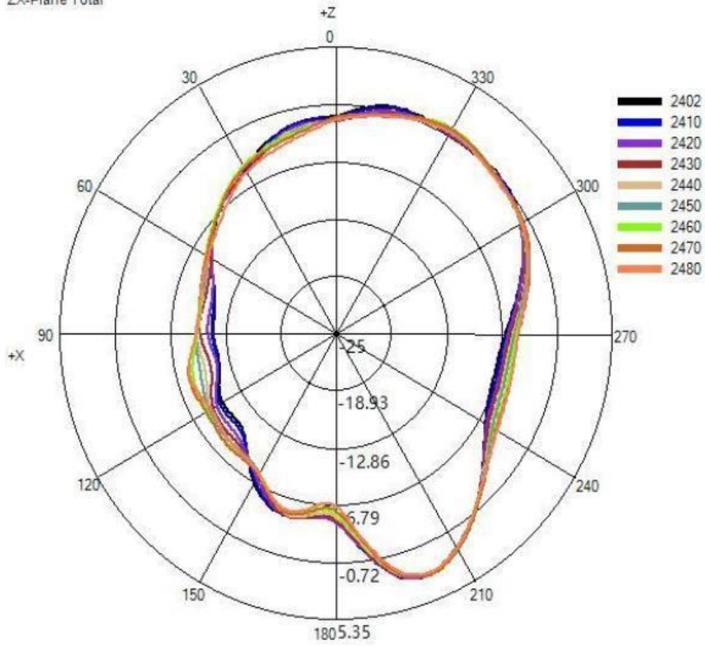
ZX-Plane Total
