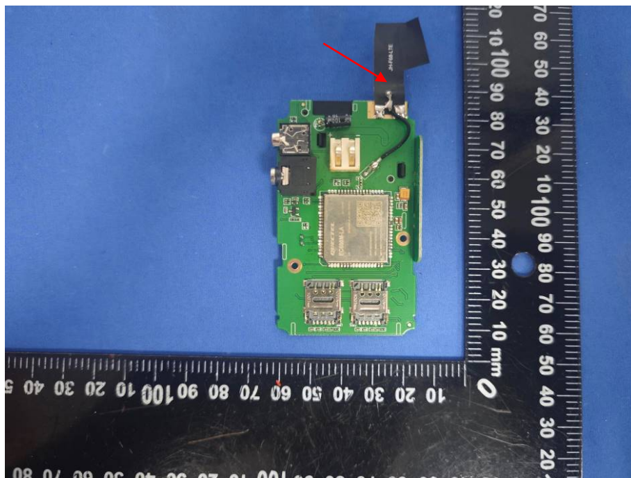
4G Antenna
