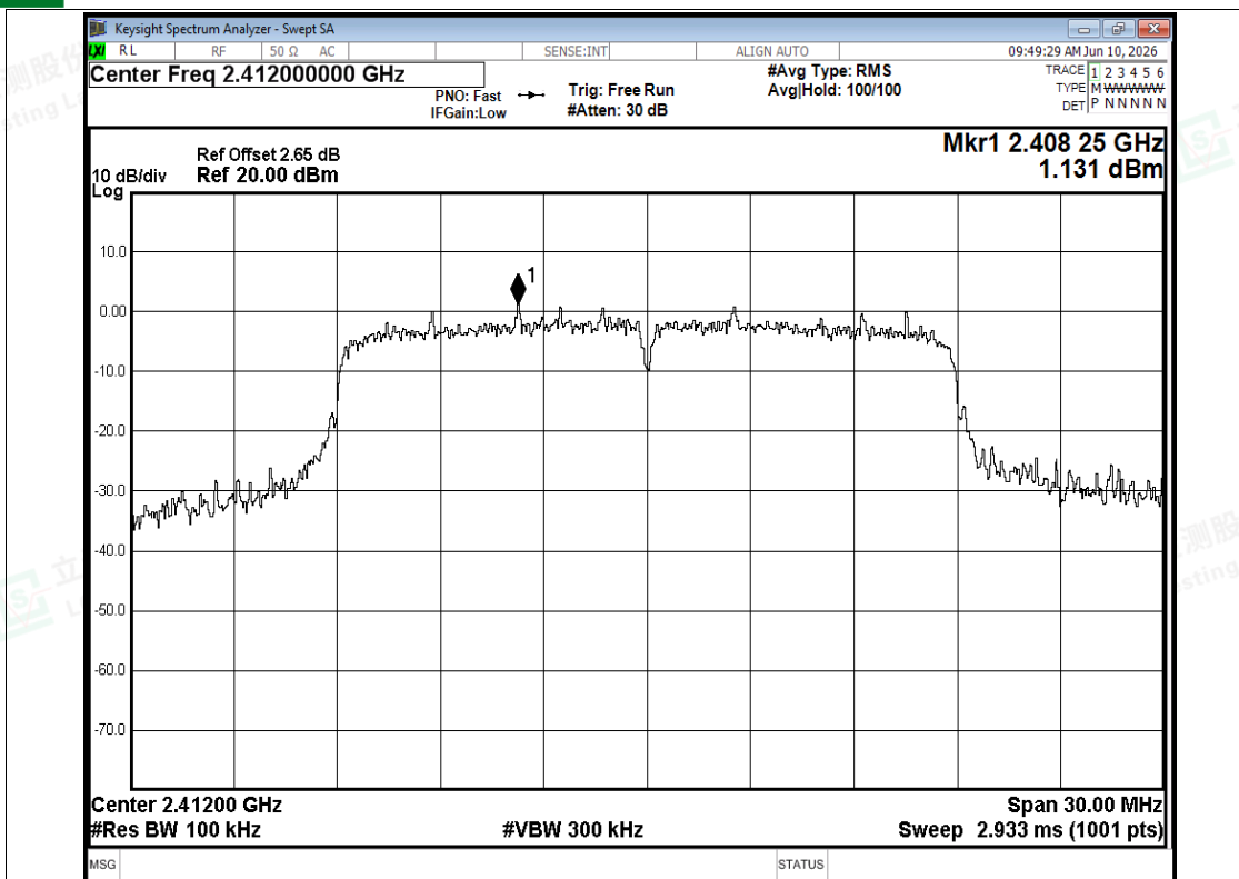
Band Edge NVNT n20 2412MHz Ant1 Ref
