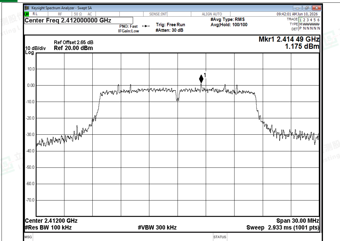
Band Edge NVNT g 2412MHz Ant1 Ref
